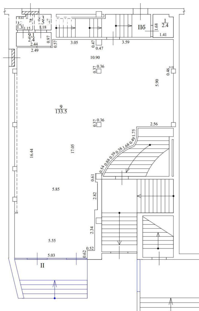
№ этажа № помещения № комнаты Назначение Площадь, кв. м 1 II 9 Помещение 133,5 9.1 Помещение 2,4 9.2 Помещение 1,3 9.3 Помещение 1,5 1 Помещение 2,4 Итого по этажу 1: 141,1
